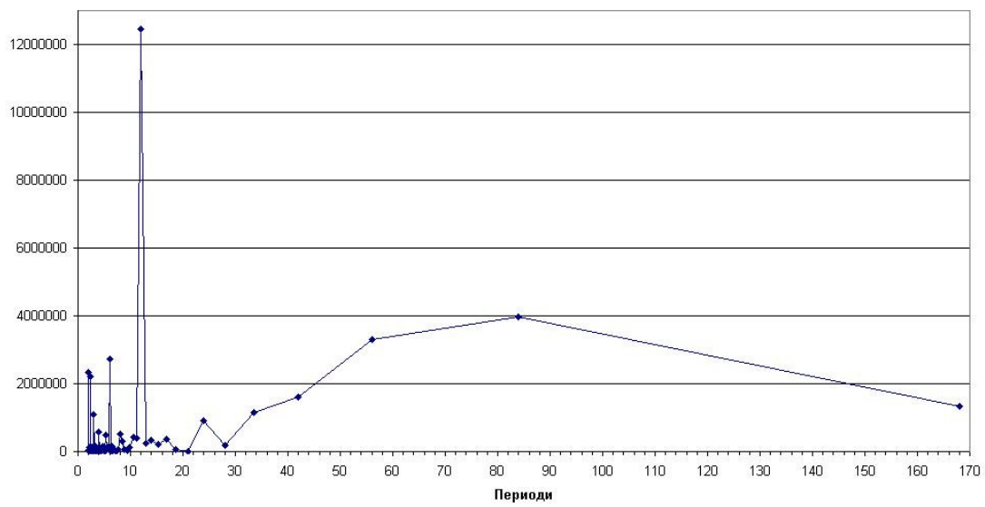
Фигура 2. Периодограма
